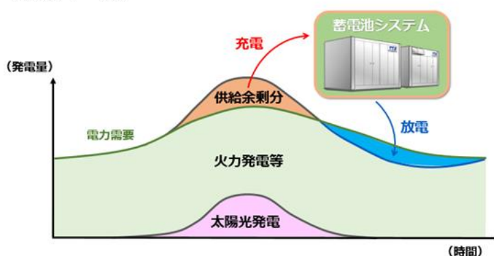
○蓄電池システムによる電力系統における課題解決例（イメージ） ①需給調整への活用
